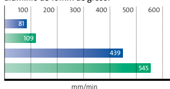
Velocidad media de soldadura para soldadura MIG y TIG manual de chapa de aleación de aluminio de 10mm de grosor
